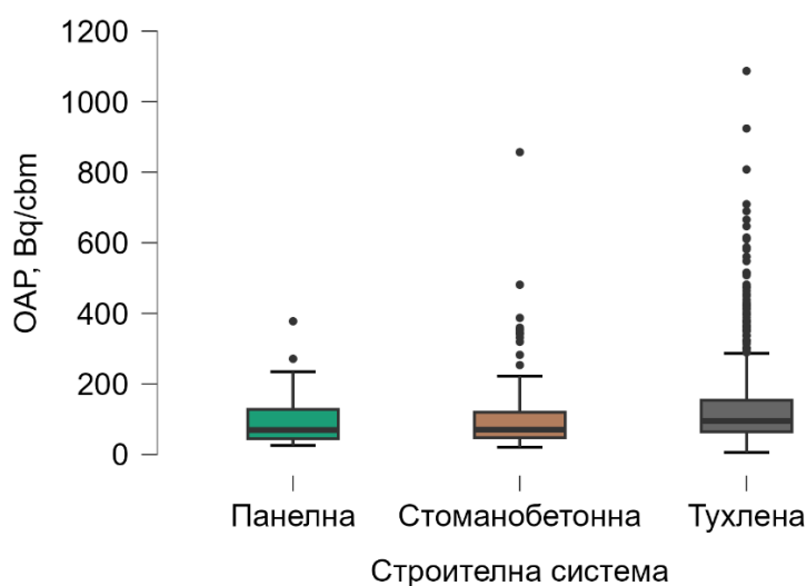
Фигура 7. Разпределение на резултатите за ОАР в [Bq/cbm] (cbm е съкращение на m 3 или кубични метра), групирани по строителна система на обследваните сгради
