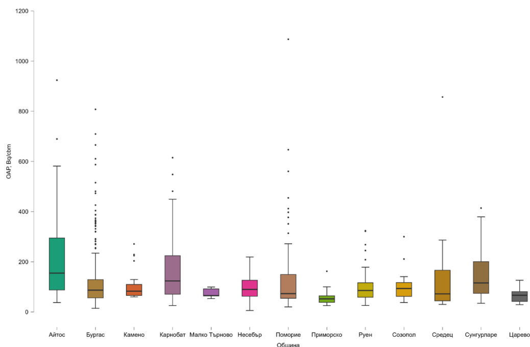
Фигура 5. Разпределение на средно аритметичната стойност на ОАР по общини
