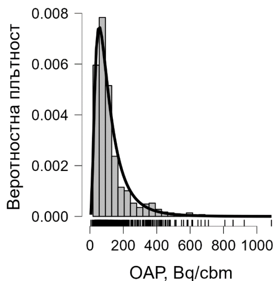
Фигура 4. Хистограма на резултатите и теоретично лог-нормално разпределение на стойностите на ОАР в [Вq/cbm] (cbm е съкращение на m^3 или кубични метра)
