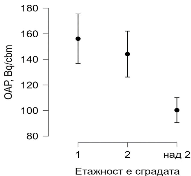
Фигура 6. Разпределение на резултатите за ОАР в [Bq/cbm] (cbm е съкращение на m^3 или кубични метра), групирани по етажност на сградите
